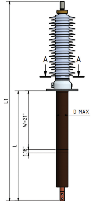
Bottom Terminal Flat Fix-conductor
